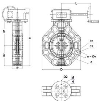
Затвор дисковый ПВХ с редуктором промышленный IPS (Model A) d8" (DN200)
