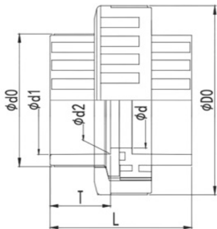
Муфта разборная ПВХ клеевая IPS d75
