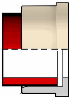
Муфтовое окончание для раструбной сварки PP-H FIP d20 PN10
