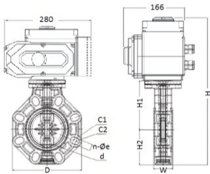
Дисковый затвор IFK ХПВХ с электрическим приводом 220V AC, EPDM, IPS d160 (DN150)
