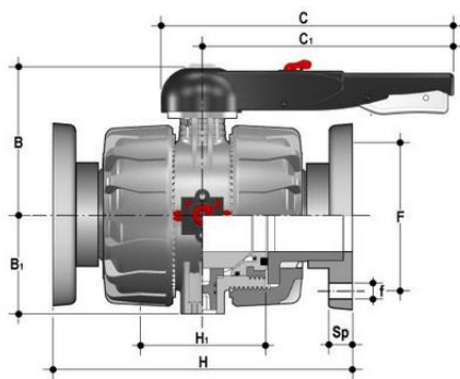
Шаровой кран промышленного применения VKD ХПВХ с фланцевыми окончаниями, DN65-100 d110 (DN90)
