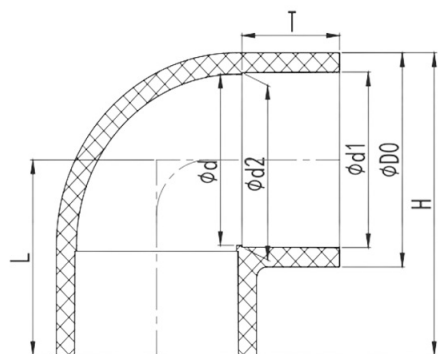
Отвод клеевой 90° ПВХ IPS d20
