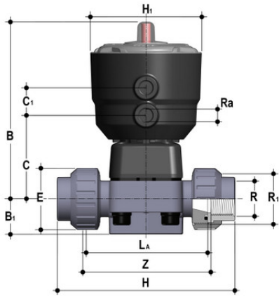
Мембранный клапан ПВХ с пневмоприводом, PN10, DK, FKM, FIP R1 1/2" (DN40)
