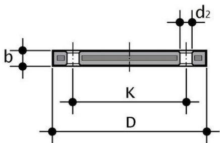
Глухой фланец PP-H FIP (PN10) d400 PN10
