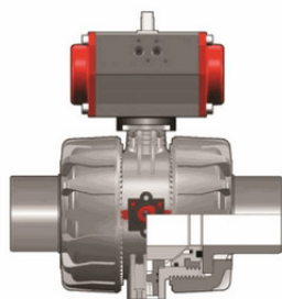
Шаровой кран VKD с пневмоприводом ДвД с втулочными окончаниями, DN65-100 (уплотнение FKM) PP-H d110 (DN100)
