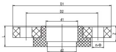
Бурт+фланец (комплект) для раструбной сварки РР-Н IPS d75 PN10
