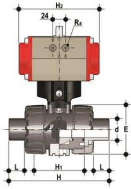
Шаровой кран VKD с пневмоприводом НО с удлинёнными патрубками из ПП (уплотнение FKM) PP-H d25 (DN20)
