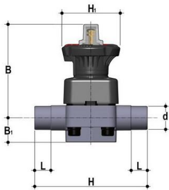
Мембранный клапан DKLDV ПВХ с муфтовыми окончаниями, EPDM, FIP d20 (DN15)
