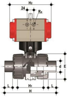
Шаровой кран VKDDVNC ПВХ с пневмоприводом НЗ с втулочными окончаниями, FKM, FIP d32 (DN25)
