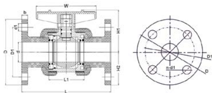
Шаровой кран IVKD ПВДФ с фланцевыми окончаниями d75 (DN65)
