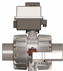
Шаровой кран VKD ПВДФ с эл.приводом 24V AC/DC, втулочные окончания d110
