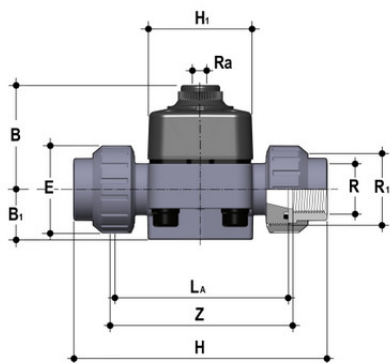
Мембранный клапан ПВХ с пневмоприводом прямого действия, DK, EPDM, FIP R3/4" (DN20)
