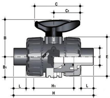
Шаровой кран промышленного применения VKD со втулочными окончаниями (уплотнение EPDM) PP-H d63 (DN50)
