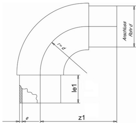
Изгиб 90° PP-H Simona (PN10) d250 SDR11 PN10
