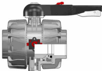
Шаровой кран промышленного применения VKD ХПВХ с муфтовыми окончаниями, DN65-100 d110 (DN90)
