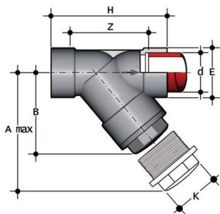
Грязевой фильтр RVIM с муфтовыми окончаниями (уплотнение EPDM) PP-H d90 (DN80)
