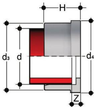
Муфтовое окончание для раструбной сварки PP-H FIP PN10
