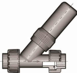
Угловой предохранительный клапан SV PBX с резьбовыми окончаниями, EPDM, FIP R3/4" (DN20)
