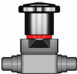
Компактный мембранный клапан CMDV PBX с втулочными окончаниями, EPDM, FIP d20 (DN15)
