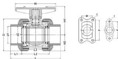
Кран шаровой ПВХ муфтовый общего применения IPS d25
