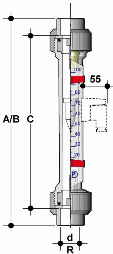
FS ротаметр для воздуха; корпус: трогамид ; поплавок с магнитом d40
