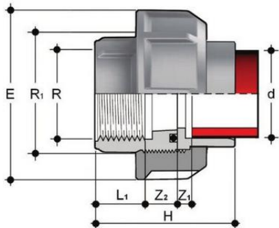
Разборная муфта с ВР, раструбная сварка РР-Н (FKM) FIP 25x3/4 PN10
