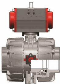
Шаровой кран VKD ПВХ с пневмоприводом НЗ с муфтовыми окончаниями, EPDM, FIP d75 (DN65)
