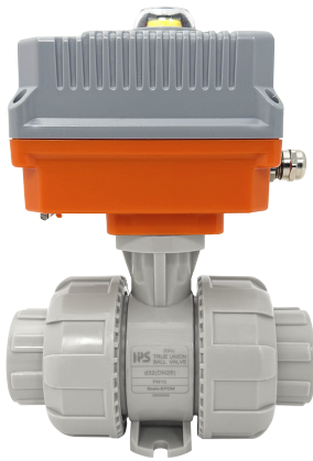
Шаровой кран IVKD ПП-гомополимер с эл.приводом 24V DC, муфтовые окончания, FKM, IPS d40 (DN32)
