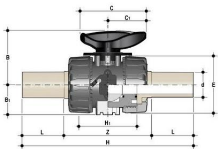
Шаровой кран для регулирования потока VKR с патрубками (CVDM) (уплотнение FKM) PP-H d50
