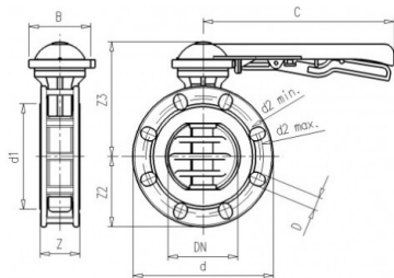
Дисковый затвор ПВХ с рукояткой, EPDM, VDL d160 (DN150)
