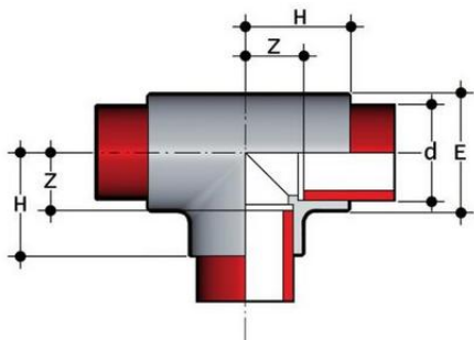
Тройник равнопроходной для раструбной сварки PP-H FIP d90 PN10
