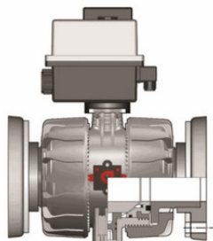
Шаровой кран промышленного применения VKD ПБХ с электроприводом, FIP d110 (DN90)
