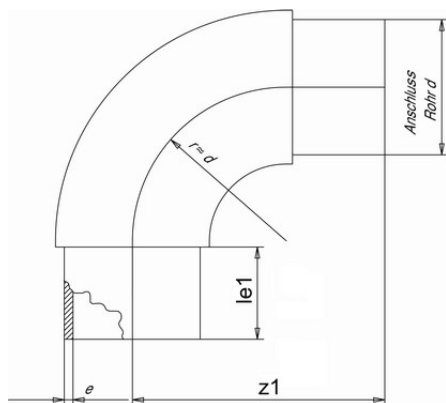
Изгиб 90° PP-H Simona d250 SDR11 PN6
