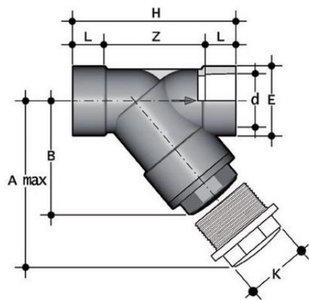
Грязевый фильтр RVIT PBX с муфтовыми окончаниями, EPDM, FIP d90
