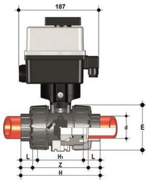
Шаровой кран для регулирования потока VKR ПВДФ с эл.приводом 24V AC 12VDC, муфтовые окончания d20 (DN15)
