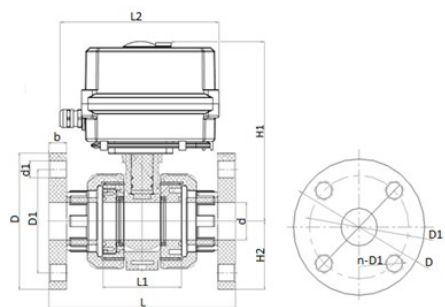
Шаровой кран IVKD ПБХ с эл.приводом 220V AC, фланцевые окончания, FKM, IPS d63 (DN50)
