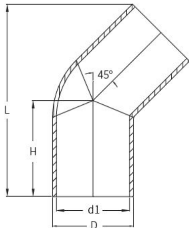
Отвод для стыковой сварки ПВДФ 45° d20 PN 16
