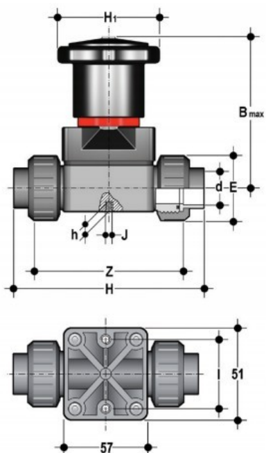
Компактный мембранный клапан CMUIC ХПВХ с втулочными окончаниями d20
