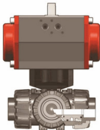
3-х ходовой шаровой кран ТКД ПБХ с пневмоприводом, L-шар, FIP d50 (DN40)
