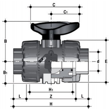
Шаровой кран промышленного применения VKD ХПВХ с муфтовыми окончаниями d16 (DN10)
