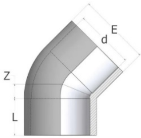
Отвод 45° ХПВХ Comer d160 PN16
