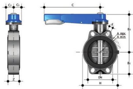
Дисковый затвор ПВХ FEOVLM с рукояткой, EPDM, FIP d160 (DN150)
