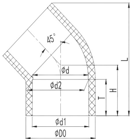
Отвод клеевой 45° ПВХ IPS d160
