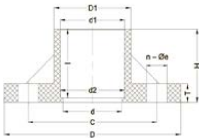
Жесткий фланец ХПВХ IPS (Model A) d50 PN16
