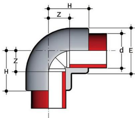
Отвод ПВДФ 90° d75 SDR21 PN16
