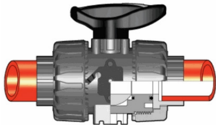
Шаровой кран промышленного применения VKD с муфтовыми окончаниями (уплотнение FKM) PP-H d40 (DN32)
