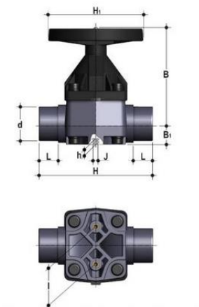
Мембранный клапан VMDV PBX с втулочными окончаниями, FKM, FIP d110 (DN100)
