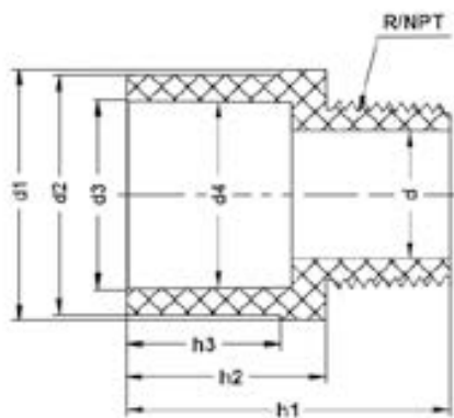
Редукционная муфта ПВДФ с НР для раструбной сварки 25х3/4" PN 16
