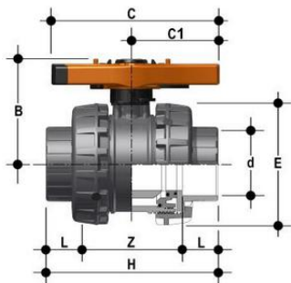
Шаровой кран общего применения VXE ХПВХ с муфтовыми окончаниями, DN65-100 d90 (DN80)
