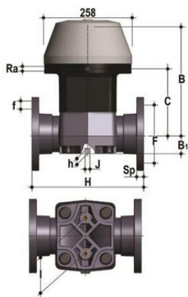
Мембранный клапан VM с пневмоприводом НЗ, PN10 с фланцевыми окончаниями (уплотнение FKM/мембрана PTFE) PP-H d90 (DN80)
